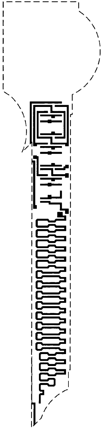
Poly mask
